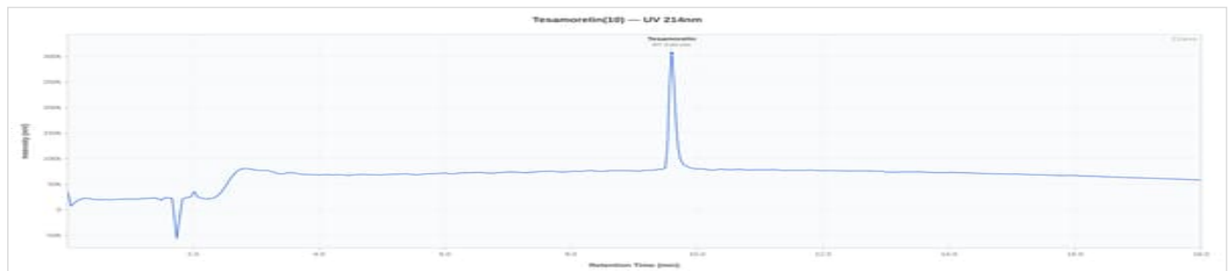
Tesamorelin 10 - PRIME1026: UV Chromatogram
